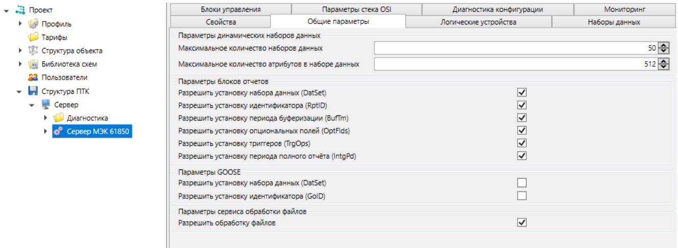
Рисунок 24 – Раздел «Общие параметры» сервера МЭК 61850
