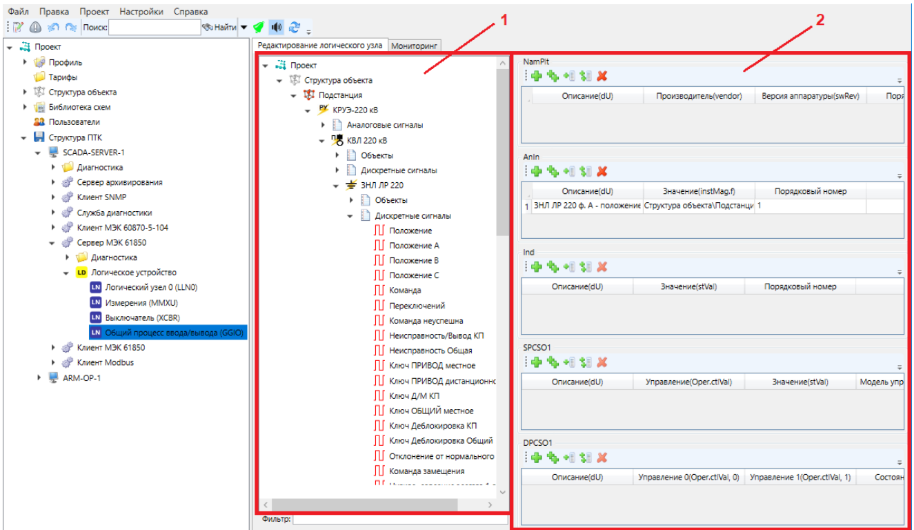
Рисунок 9 – Заполнение модели данных в сервере МЭК 61850
