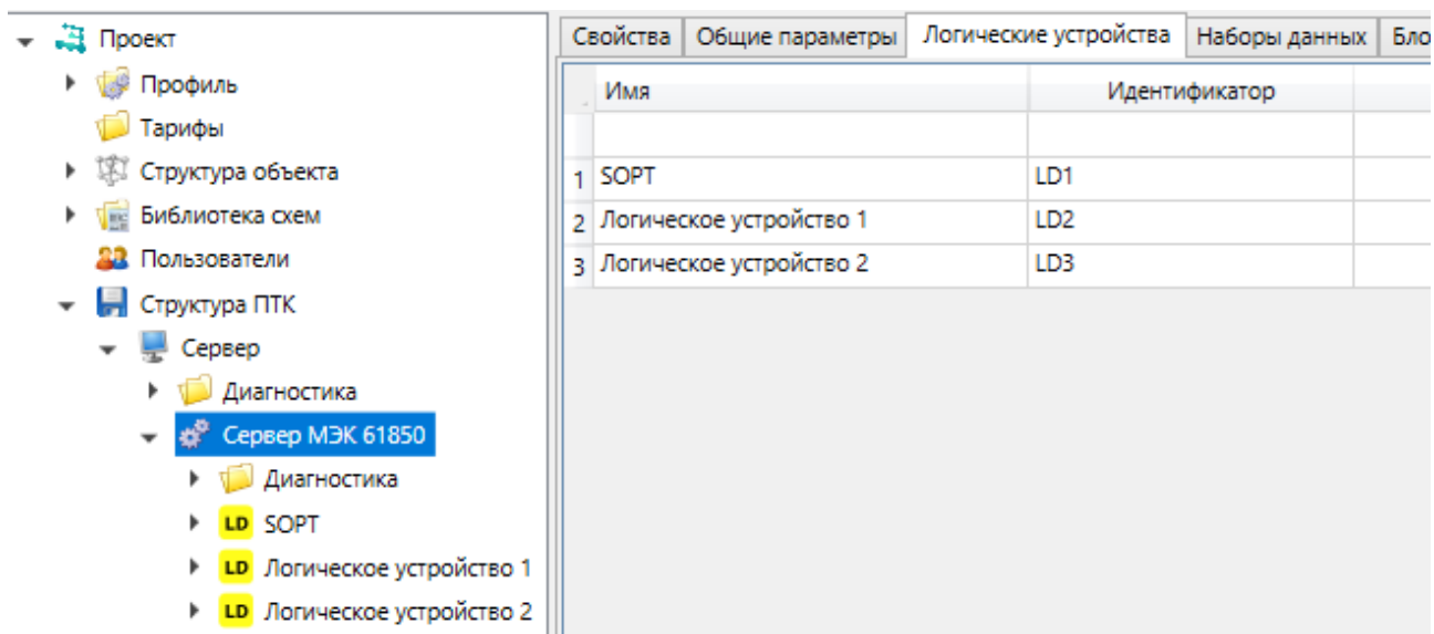
Рисунок 25 – Раздел «Логические устройства» сервера МЭК 61850
